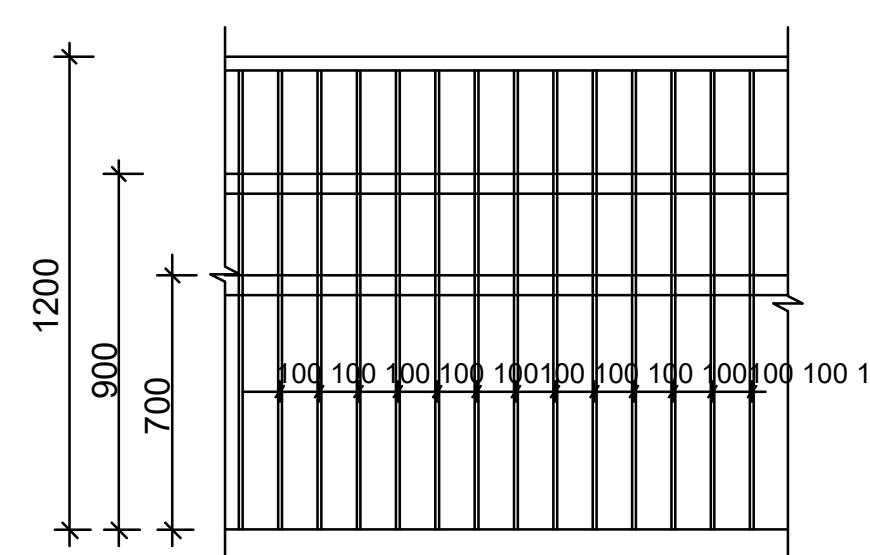
Ограждения для пандуса
