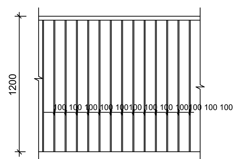
Ограждения для выходов из подвалов
