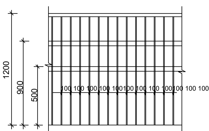
Ограждения для лестичных клеток
