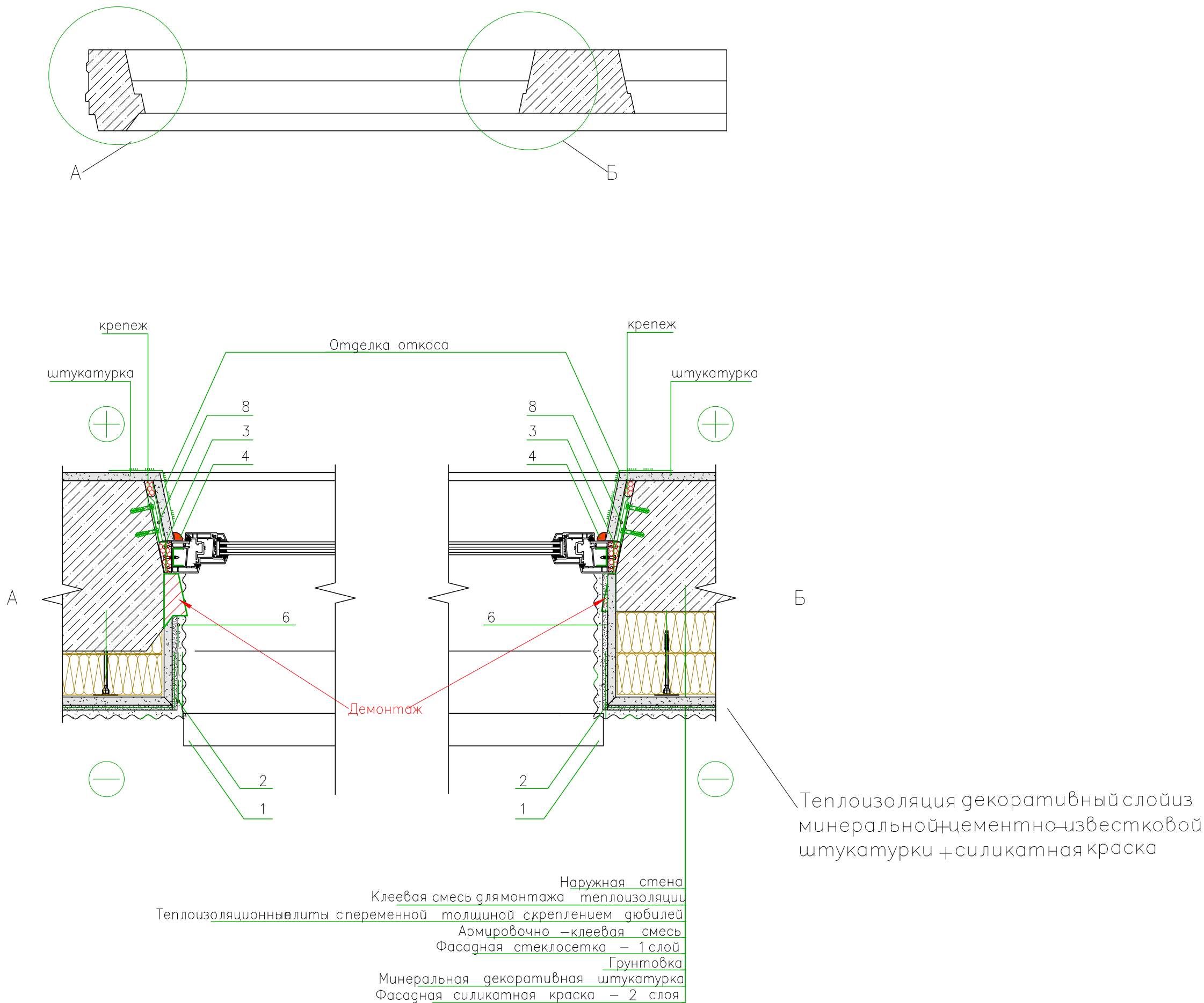
Горизонтальный разрез по оконному проему
